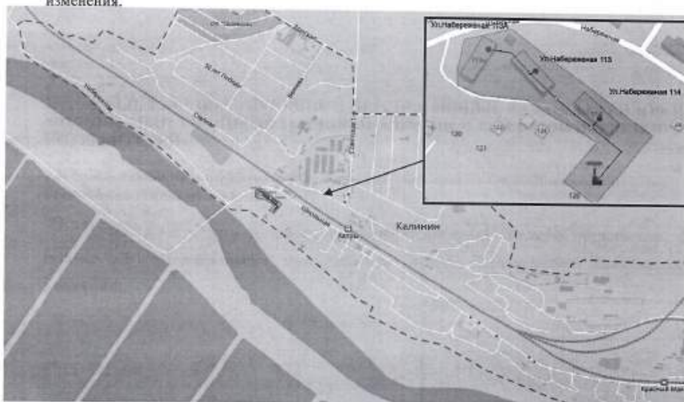
Рисунок 2.1.1 – существующие и перспективные зоны действия систем теплоснабжения и источников тепловой энергии
